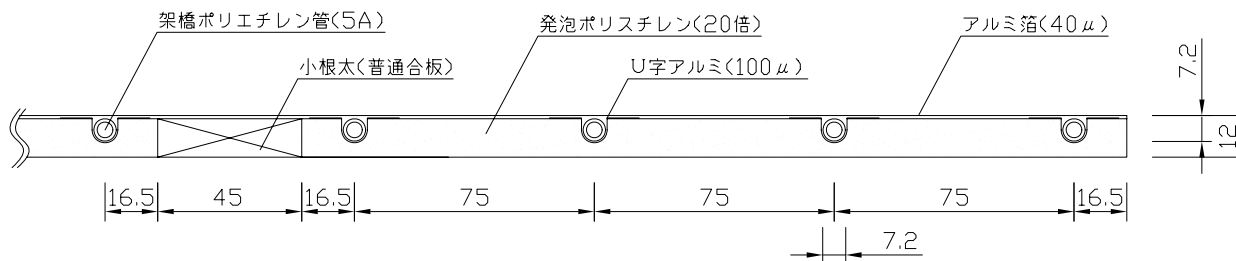
〈A-A'断面図〉
