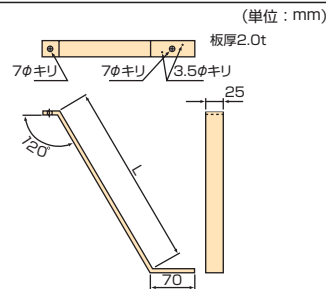
■脚(1) 寸法図
