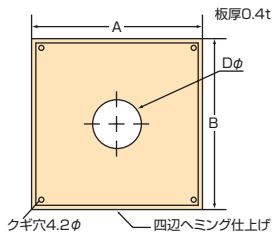
■化粧板(H) 寸法図
